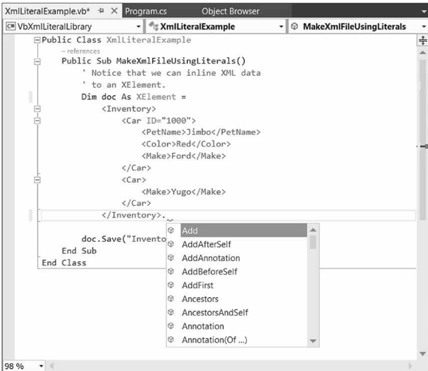
Рис. Б.1. Синтаксис литералов XML в VB представляет собой сокращение для работы с объектной моделью LINQ to XML
