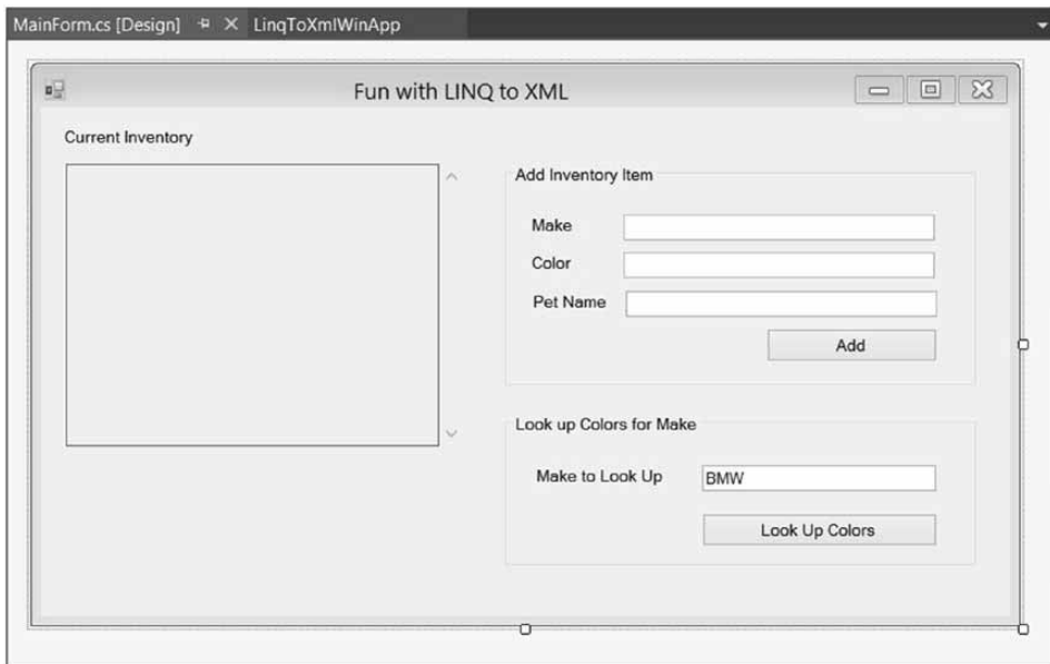
Рис. Б.4. Графический пользовательский интерфейс для приложения LINQ to XML
